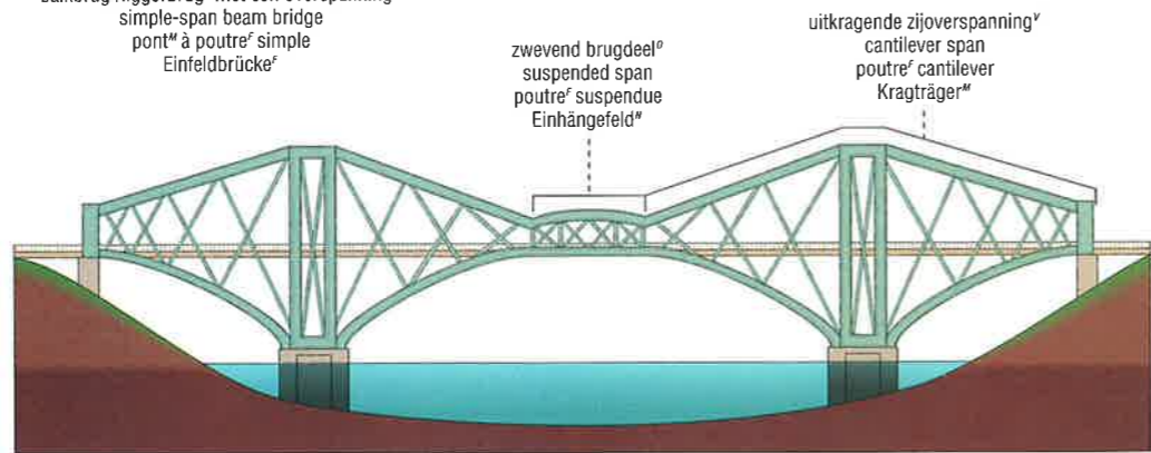
kraagliggerbrug v /cantileverbrug v cantilever bridge pont m cantilever Auslegerbrücke f
