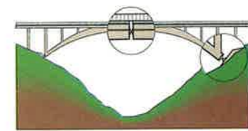
driescharnierboog m three-hinged arch arc m à trois articulations m dreiteiliger Bogen m
