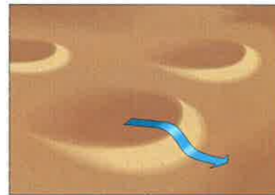
paraboolduin parabolic dune dune parabolique Parabeldüne
