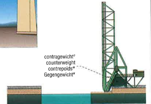
ENKELE BASCULEBRUG v SINGLE-LEAF BASCULE BRIDGE PONT m BASCULANT À SIMPLE VOLÉE f KLAPPBRÜCKE f
