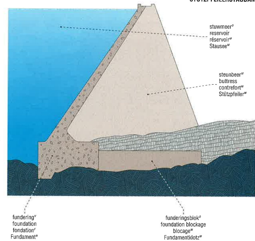
DWARSDOORSNEDE VAN EEN PIJLERSTUWDAM m CROSS SECTION OF A BUTTRESS DAM COUPE f D'UN BARRAGE m À CONTREFORTS m STÜTZPFILERSTAUDAMM m IM QUERSCHNITT m
