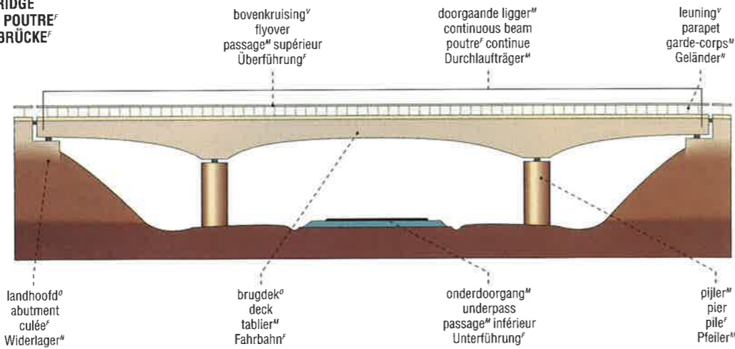
balkbrug v /liggerbrug v met meer overspanningen v multiple-span beam bridge pont m à poutres f indépendantes Mehrfeldbrücke f
