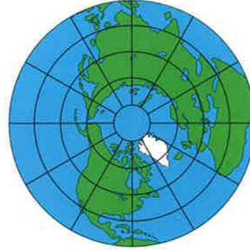
azimutale projectie plane projection projection horizontale Azimutalprojektion
