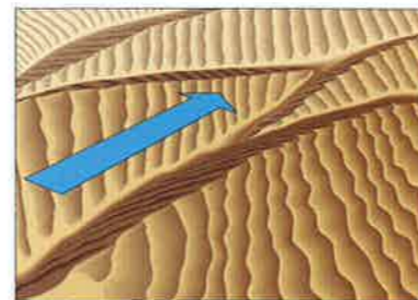
lengteduinen longitudinal dunes dunes longitudinales Längsdünen
