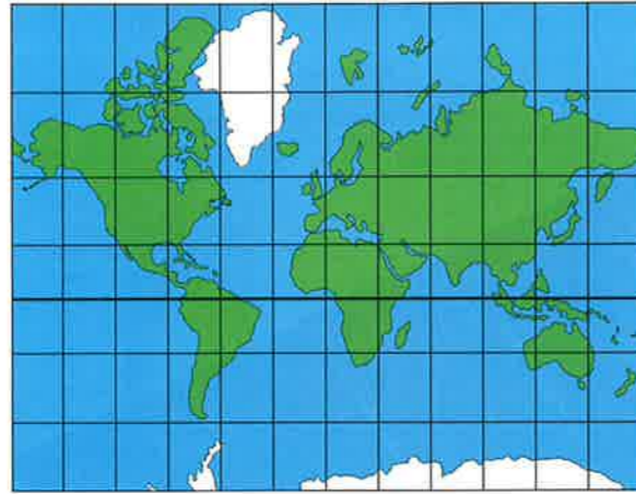
cilinderprojectie cylindrical projection projection cylindrique Zylinderprojektion
